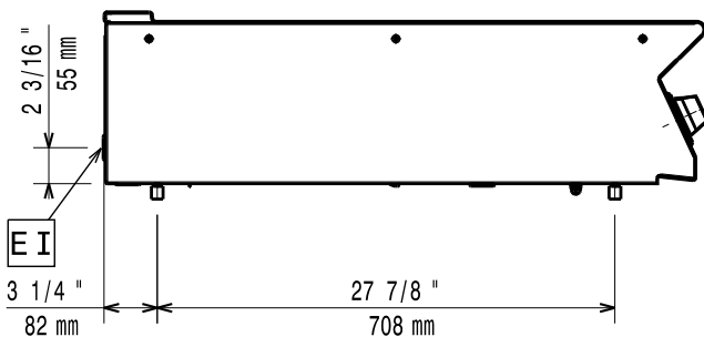
Zij aanzicht
