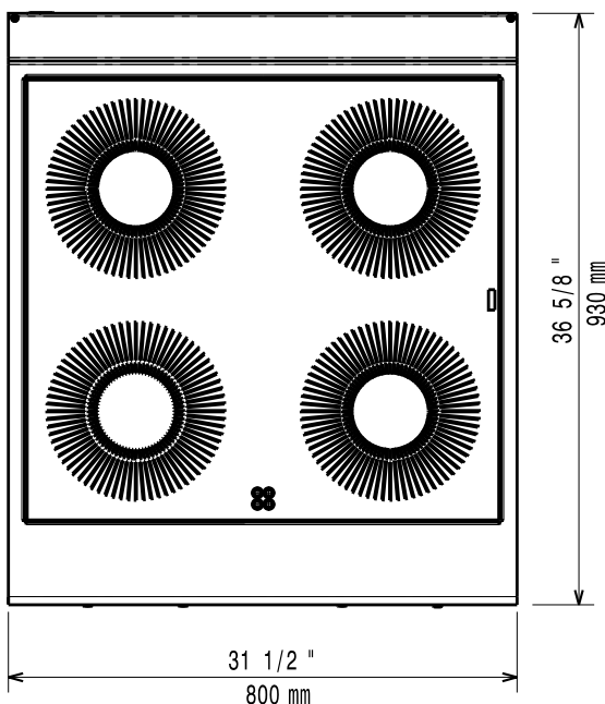
Boven aanzicht
